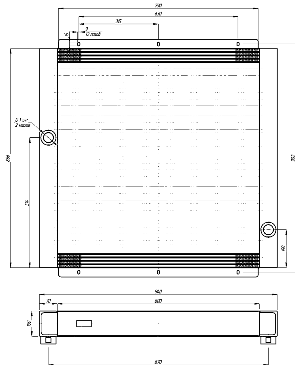
Рисунок 8. Охладитель масла.
