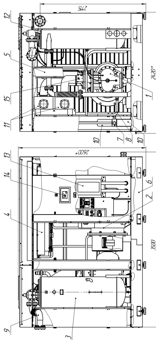
Рисунок 2. Установка компрессорная.
