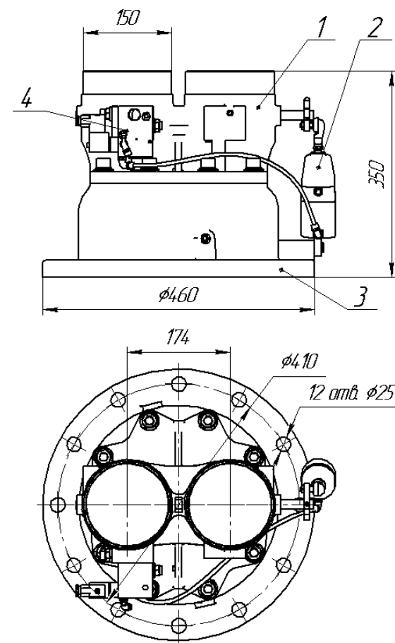
исунок 4.Клапан впускной.
