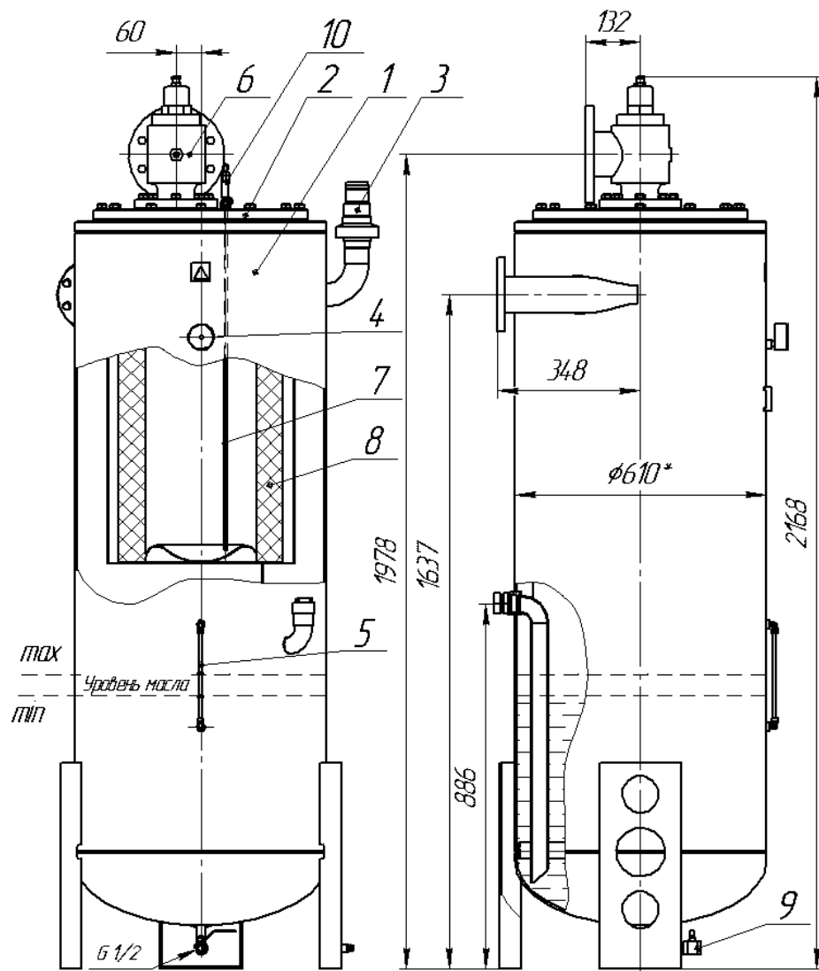
Рисунок 5. Маслоотделитель.
