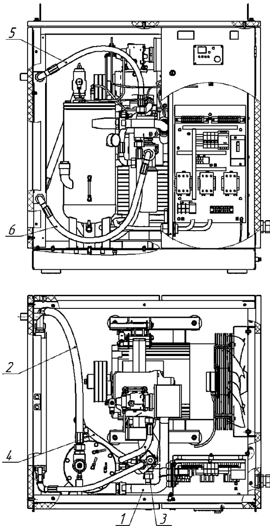
Рисунок 11. Схема расположения рукавов.
