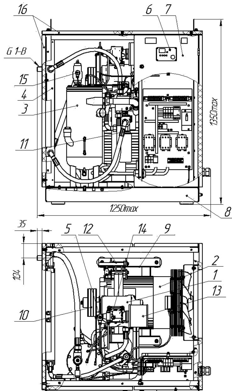
Рисунок 2. Установка компрессорная.
