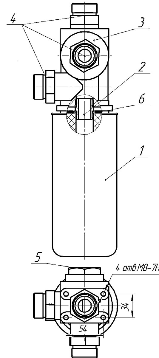
Рисунок 8. Блок распределения.
