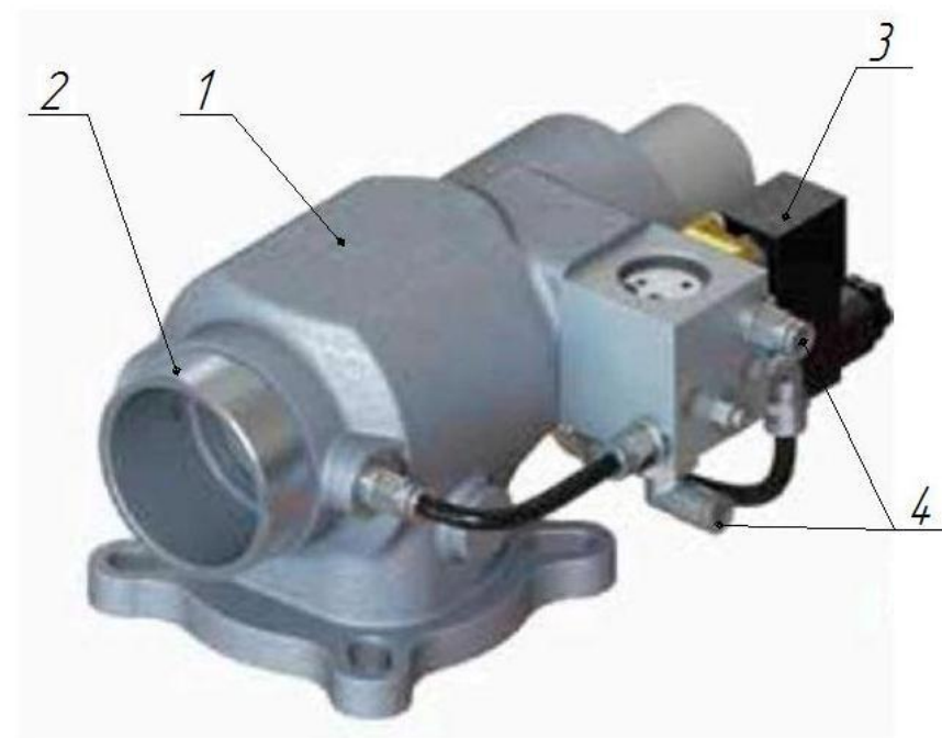
Рисунок 4. Клапан впускной.
