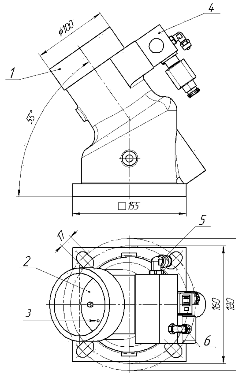
Рисунок 4. Клапан впускной.
