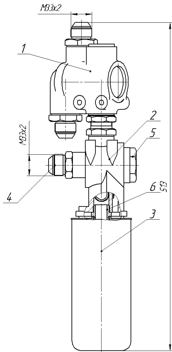
Рисунок 7. Блок распределения.
