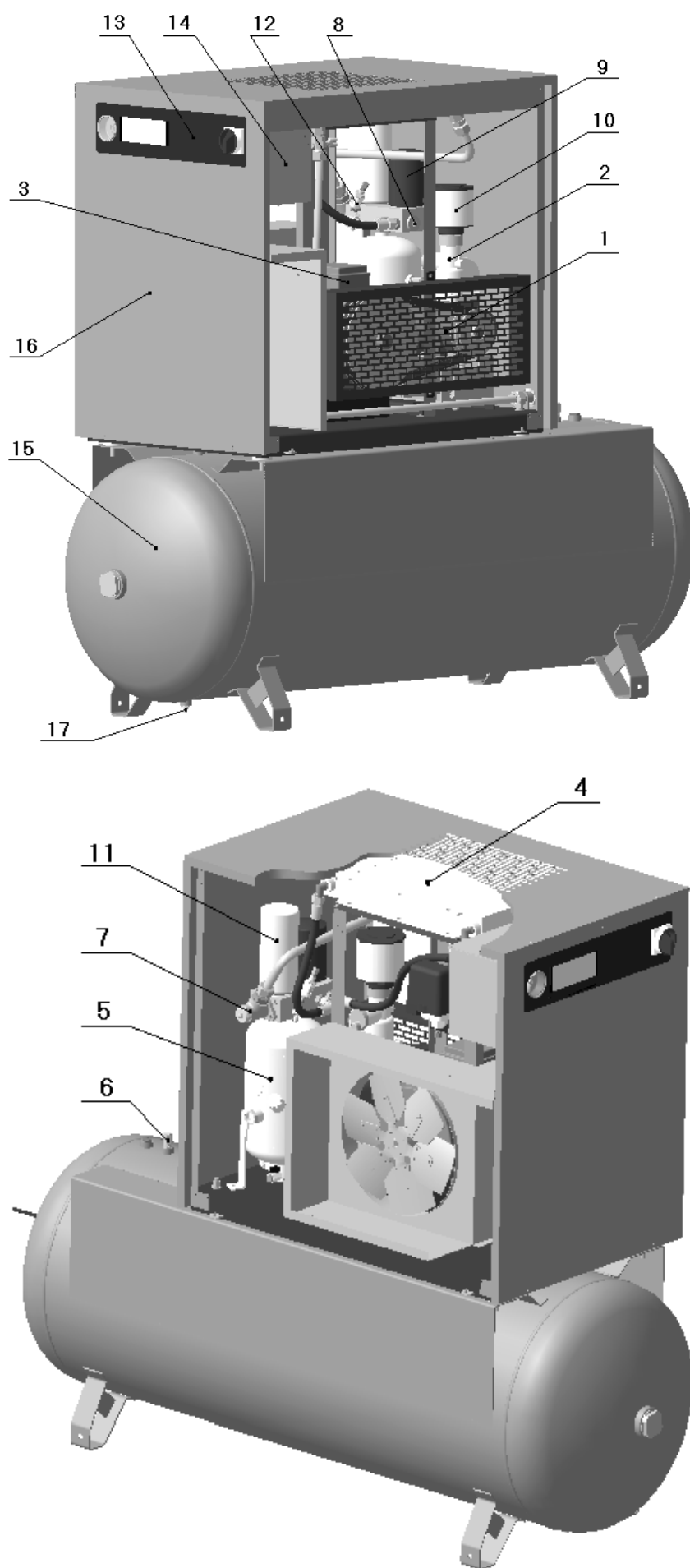
Рисунок 2 – Общий вид компрессорной установки BK15E-...-500
