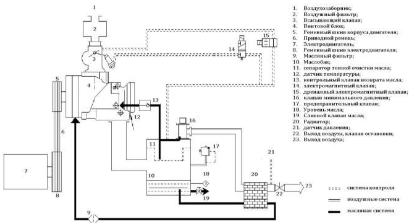
Технологическая схема компрессора ВК-11 и более мощных моделей
