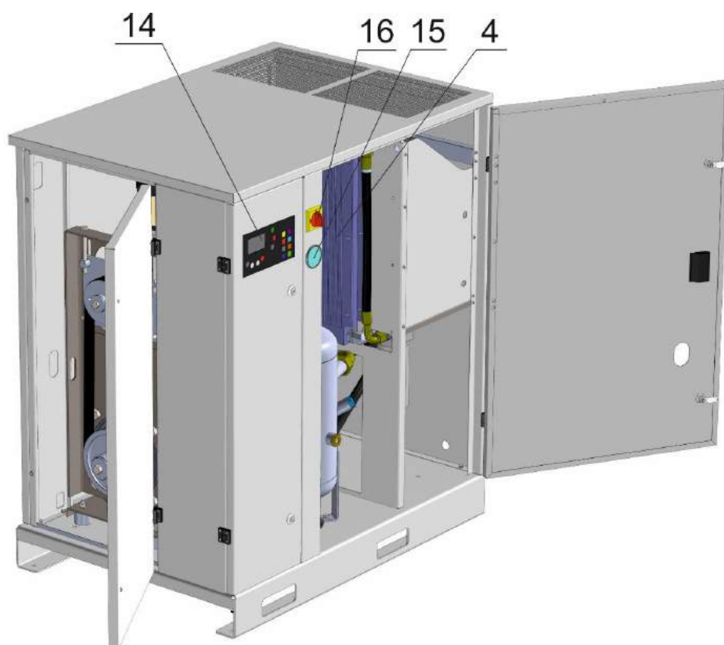
Рисунок 1 – Общий вид компрессорной установки ВК25Т-...(ВС), 30Т-...(ВС)
