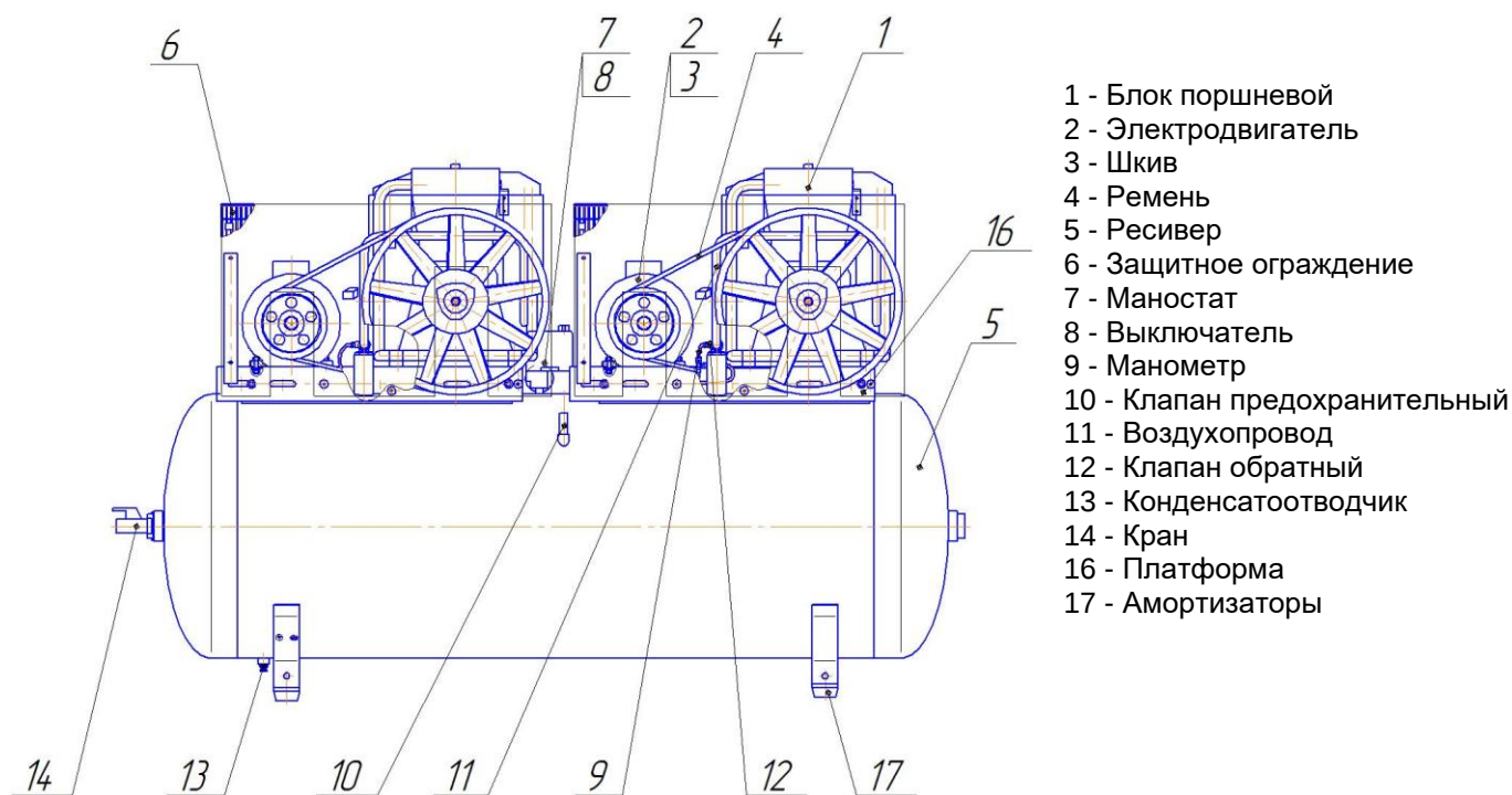
Рисунок 4 - Общий вид компрессора АБТ 500-2200 WB
