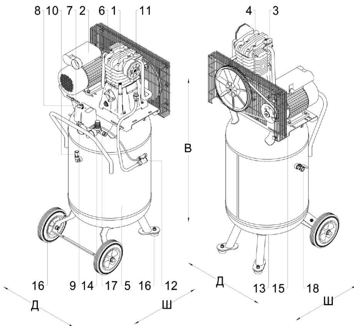
Рисунок 8 - Общий вид компрессора СБ4/С-100.АВ365В(АВ)(470В)
