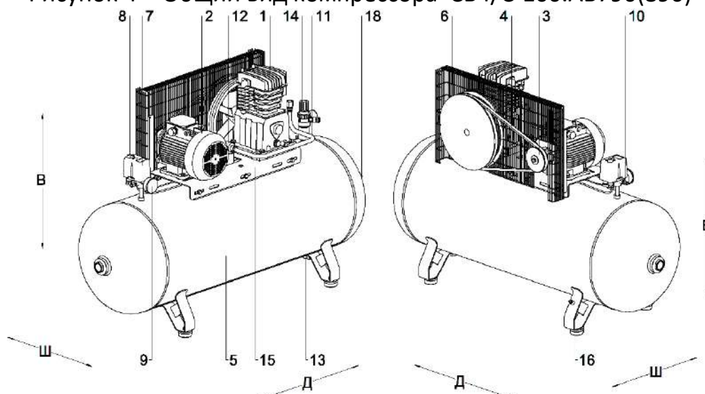
Рисунок 5 - Общий вид компрессора СБ4/Ф-270.АВ890
