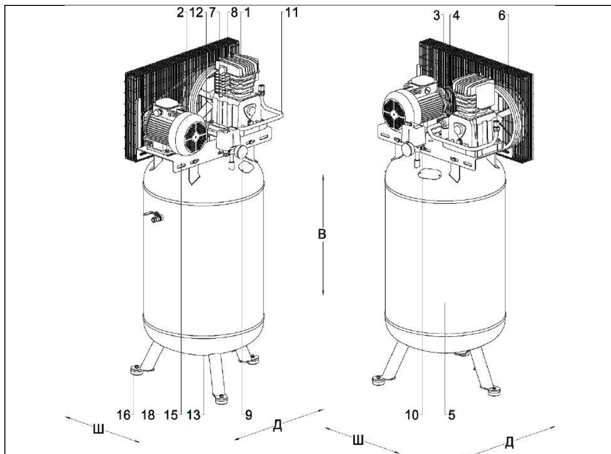
Рисунок 6 - Общий вид компрессора СБ4/Ф-270.АВ790(890)В
