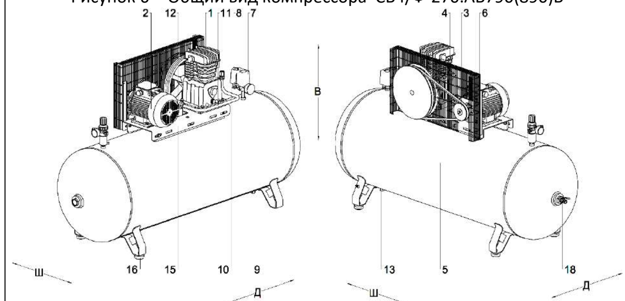
Рисунок 7 - Общий вид компрессора СБ4/Ф-50.АВ890
