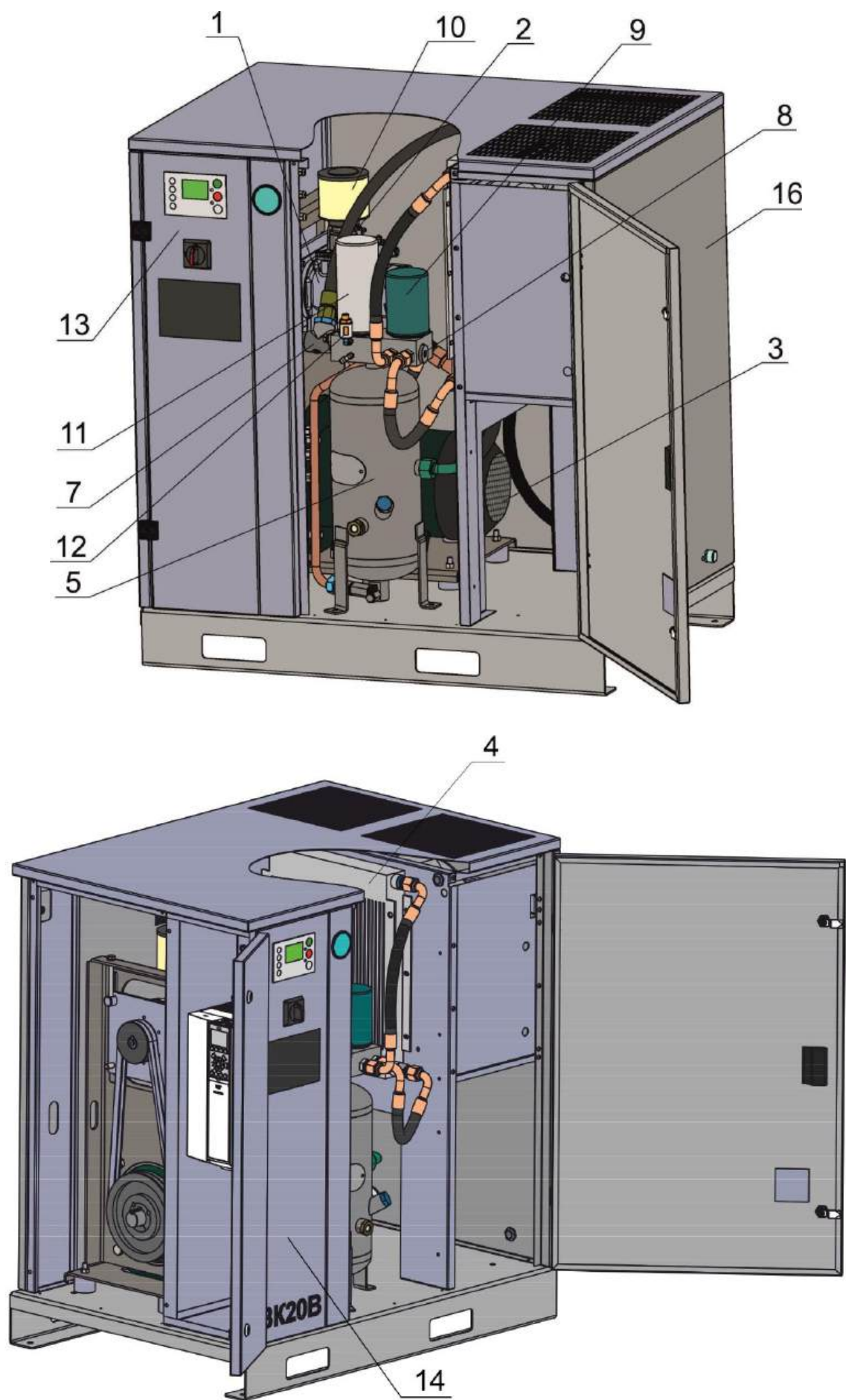
Рисунок 1а – Общий вид компрессорного агрегата установки ВК15Т-16-500Д2
