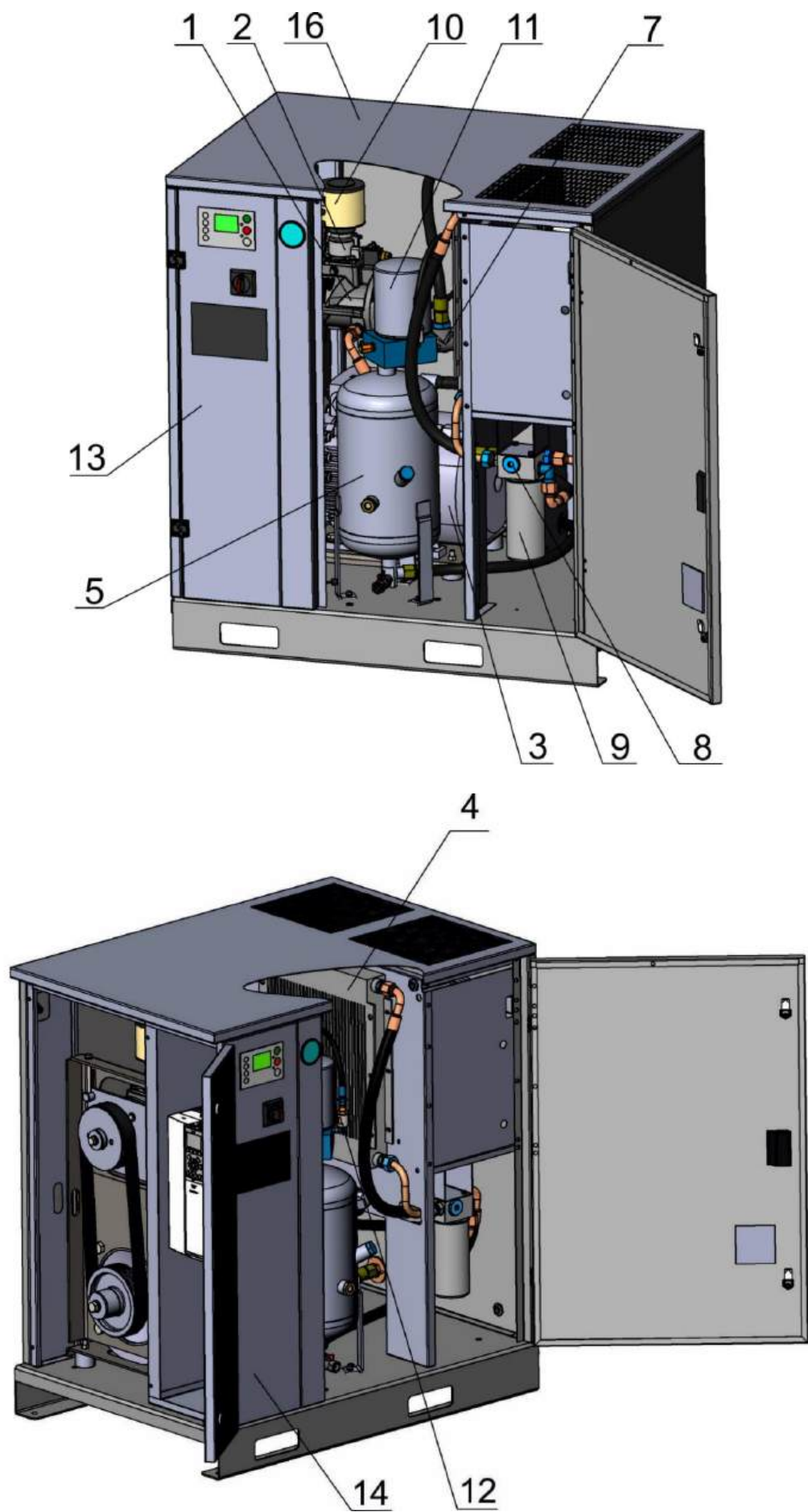
Рисунок 16 – Общий вид компрессорного агрегата установки ВК20Т-16-500Д2
