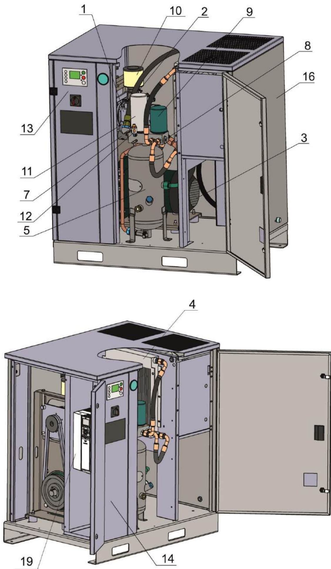
Рисунок 1 – Общий вид компрессорной установки ВК20Т-...(BC)
