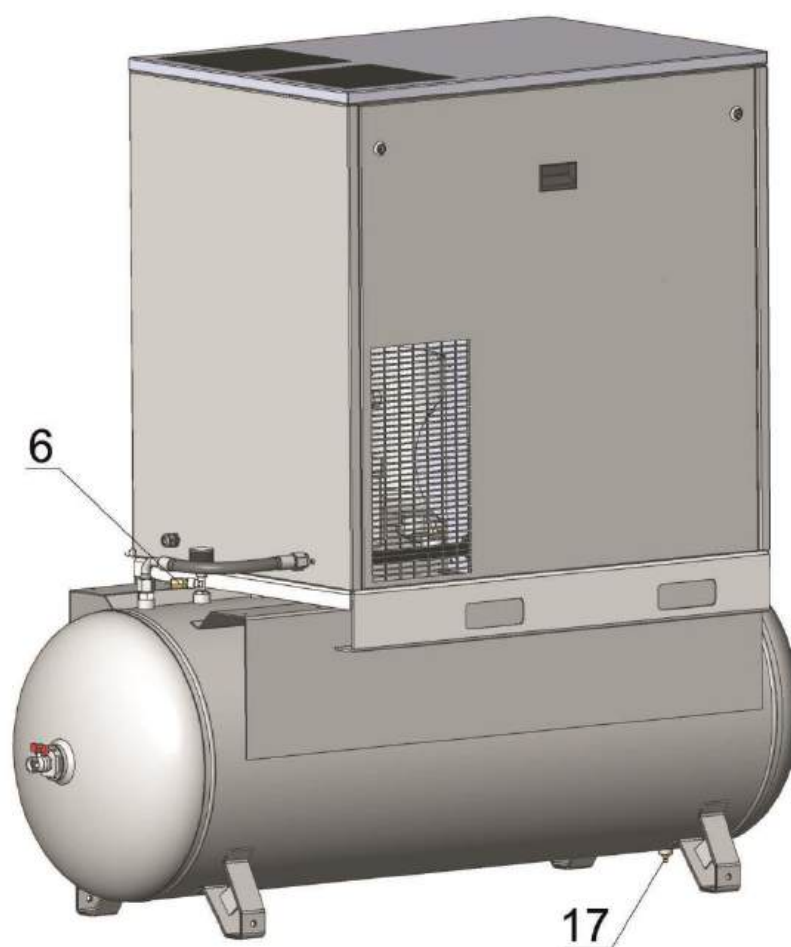
Рисунок 2 – Общий вид компрессорной установки ВК20Т-...-500(ВС)
