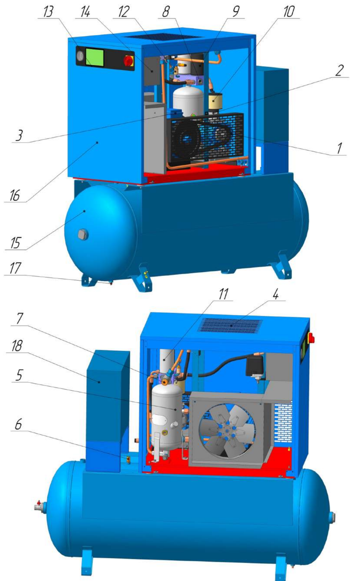
Рисунок 3 – Общий вид компрессорной установки ВК15Т-...-500Д
