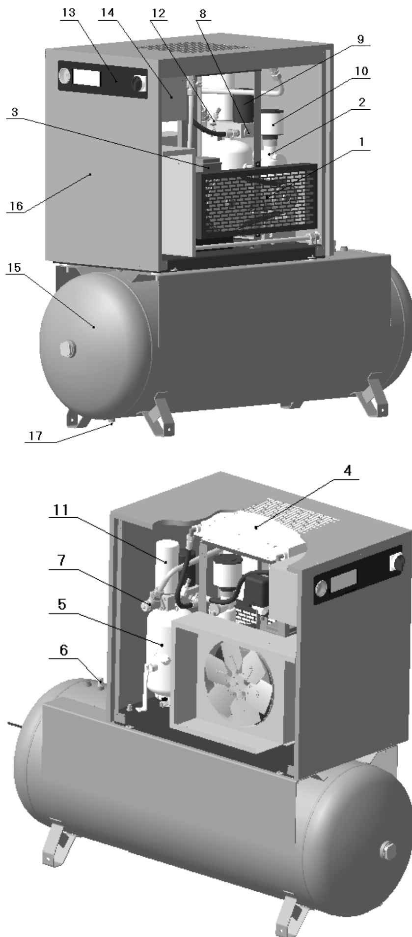
Рисунок 2 – Общий вид компрессорной установки VK15T-...-500
