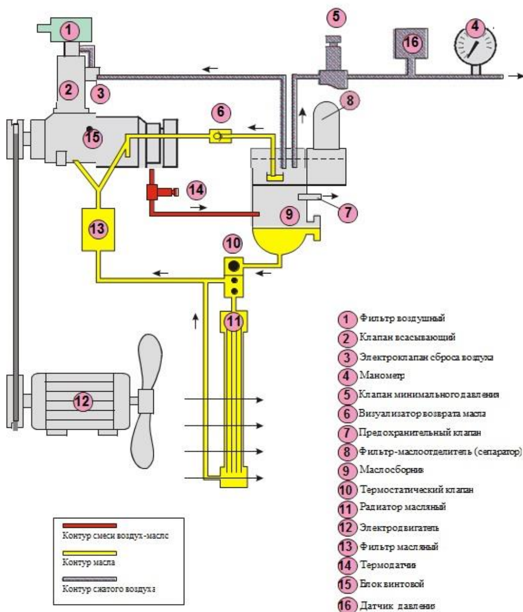
Рисунок 4 – Схема функциональная принципиальная компрессорных установок BK5T, BK7T, BK10T
