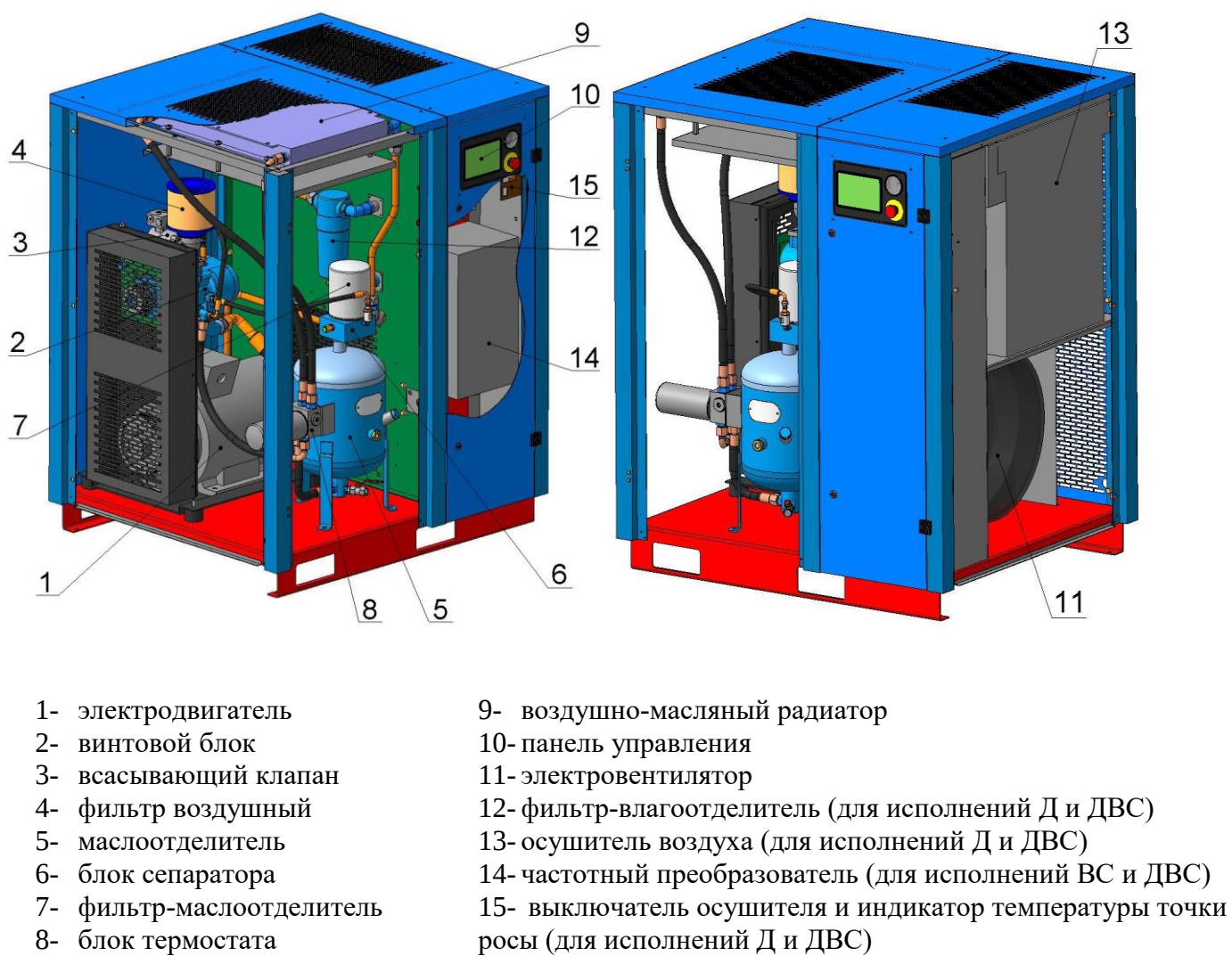
Рисунок 2 – Основные узлы компрессорной установки
