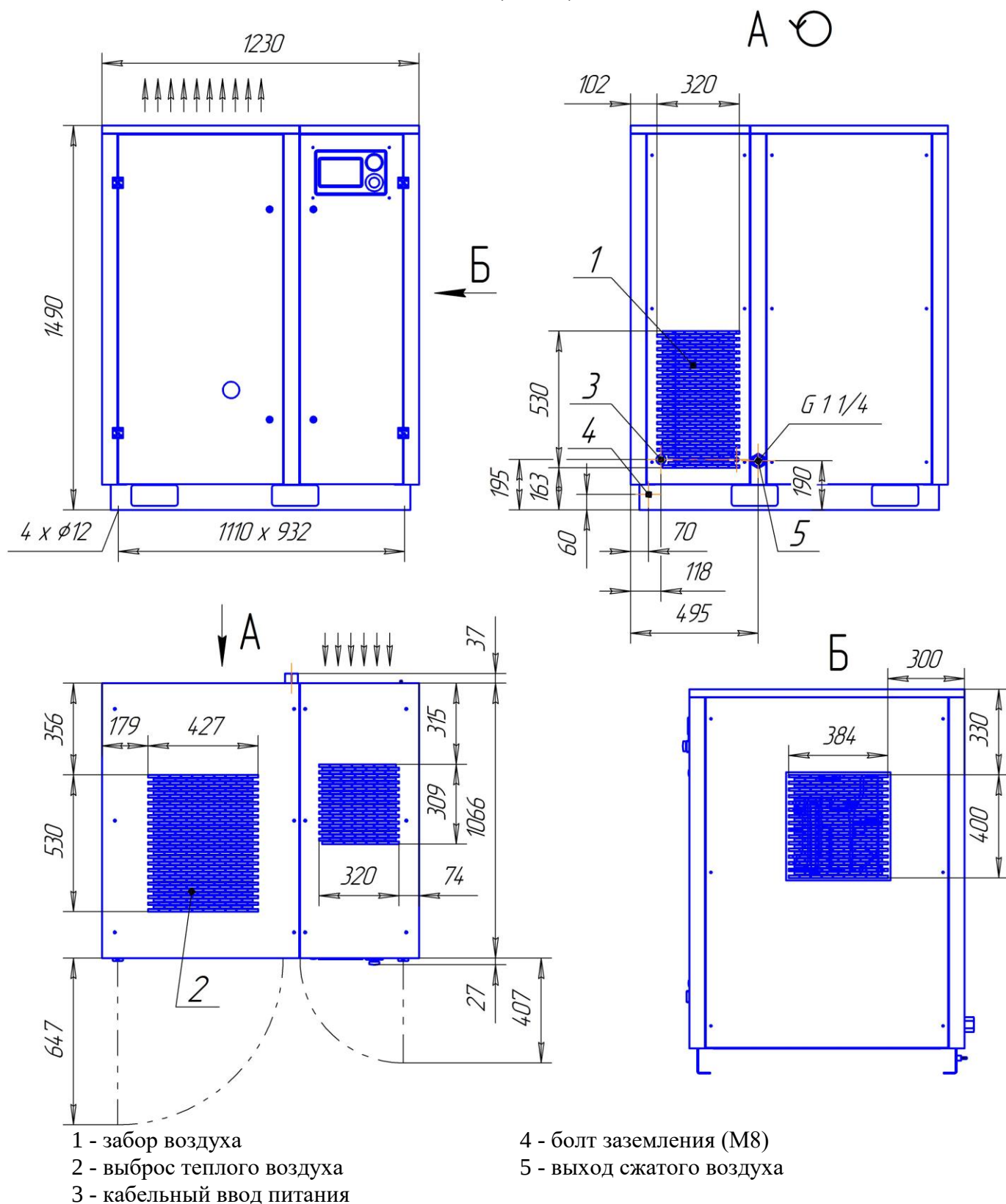
Рисунок А.1 – Присоединительные и установочные размеры компрессорной установки
