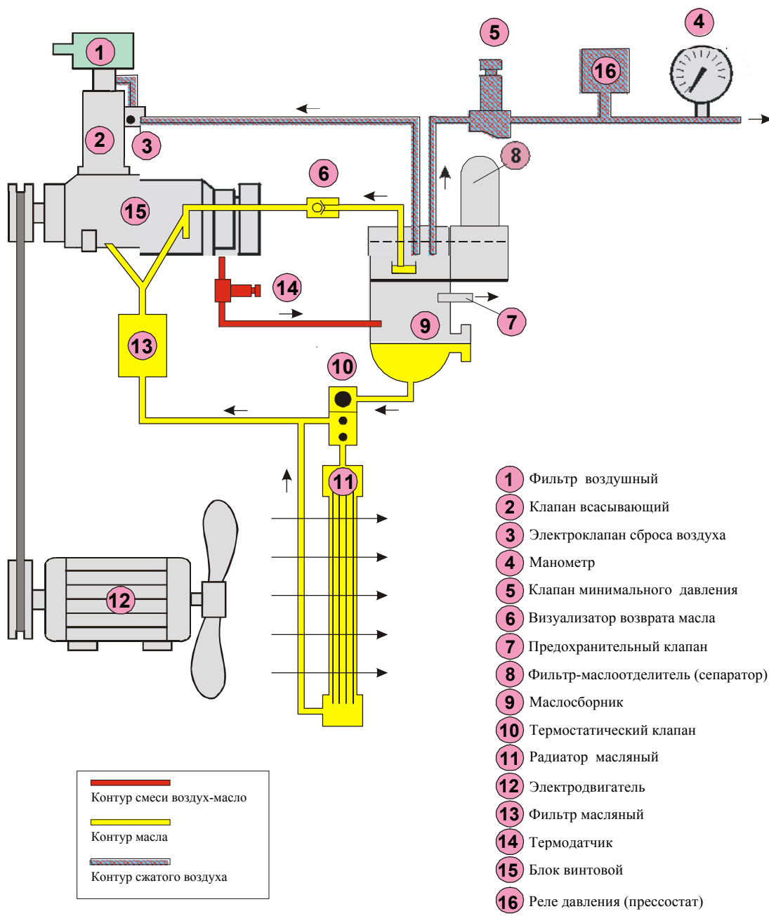
Рисунок 4 – Схема функциональная принципиальная компрессора ВК5, ВК7, ВК10
