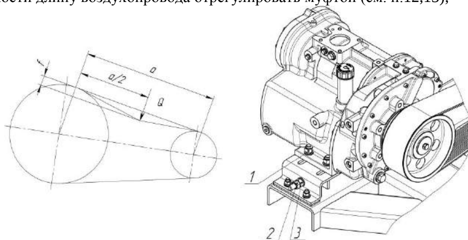
Рис. 4а. Натяжение ремня CG80 / CS80.
