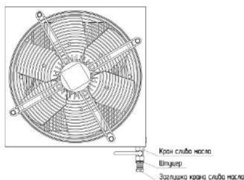
Рис. 6. Маслоохладитель
