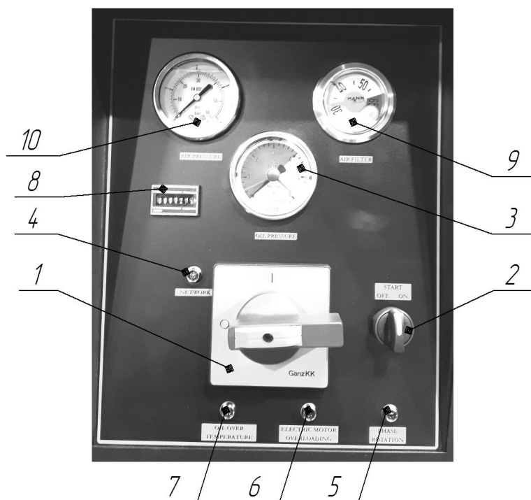
Рис. 3. Панель управления
