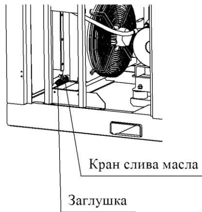
Рис. 6. Маслоохладитель
