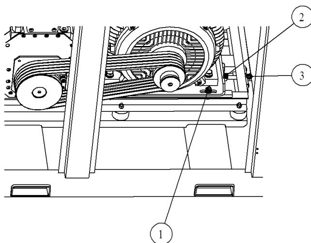
Рис.4 Натяжение ремней
