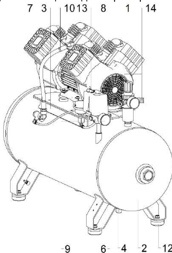
Рисунок 5 - Общий вид компрессора СБ4/Ф-100.4V55
