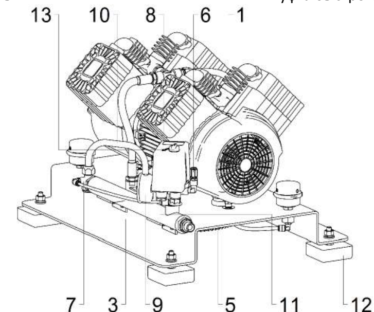
Рисунок 4 - Общий вид компрессора СБ4-4V55
