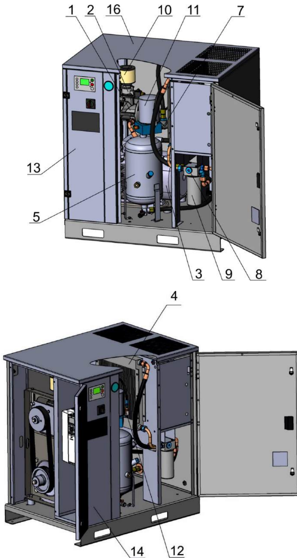
Рисунок 1 – Общий вид компрессорной установки ВК20Е-8(10, 15)
